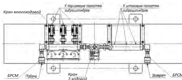
Шаровый кран 2-ходовой. Предназначен для аварийного сброса гидравлической жидкости из напорной в сливную магистраль
