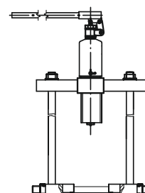
Вариант сборки с хомутом
