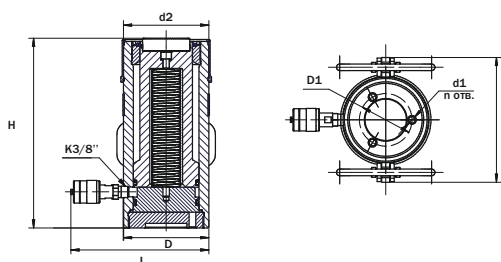
Модели: ДУ20П50, ДУ35П50, ДУ100П50, ДУ100П150
