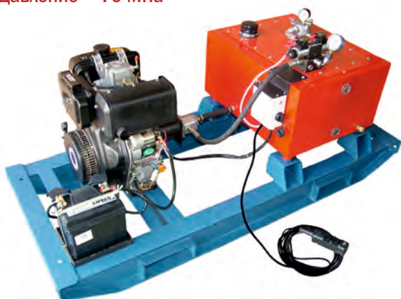
Модель: НДЭ-10К100-1-П10 с пультом 10м
