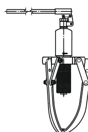
Вариант сборки с лапами
